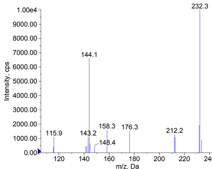
+ 5F-ADBICA Prec(362.0) CE(50.0) RT(0.3)
