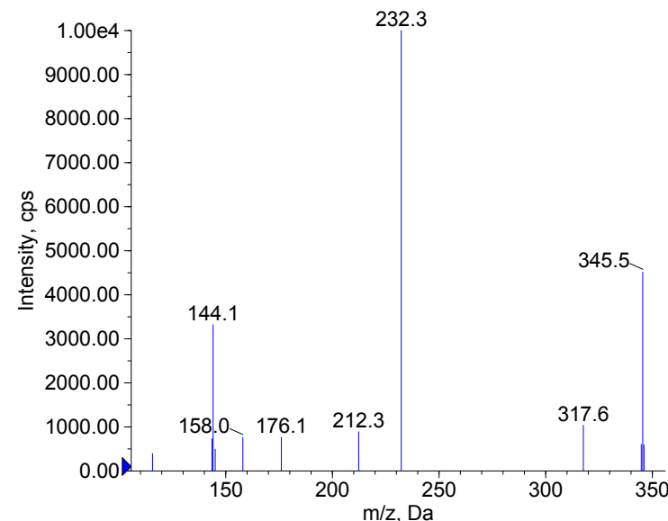
+ 5F-ADBICA Prec(362.0) CE(99.0) RT(0.3)
