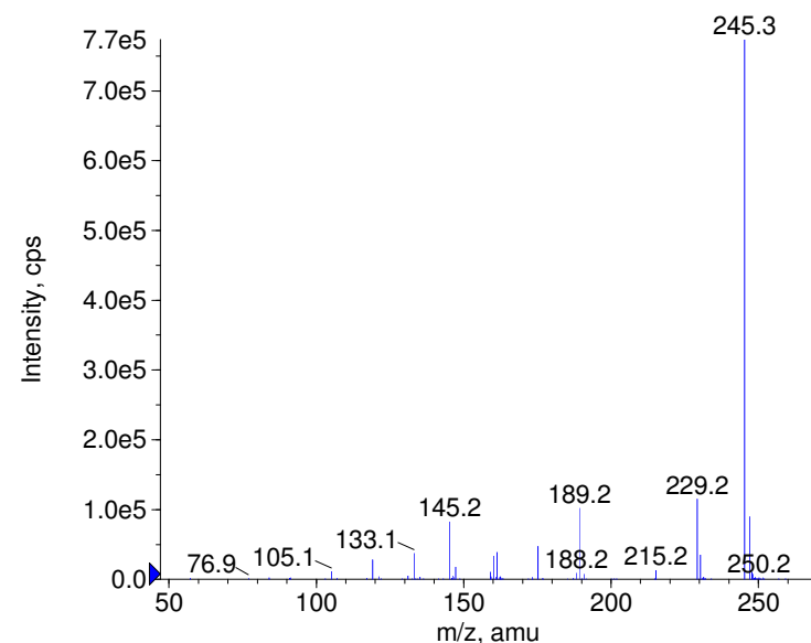
+ Xylometazoline Prec(245.0) CE(99.0) RT(0.9)
