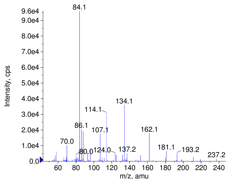
+ Xantinol Prec(312.0) CE(50.0) RT(0.9)
