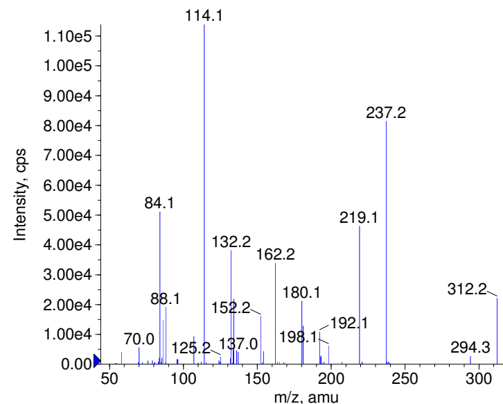
+ Xantinol Prec(312.0) CE(99.0) RT(0.9)
