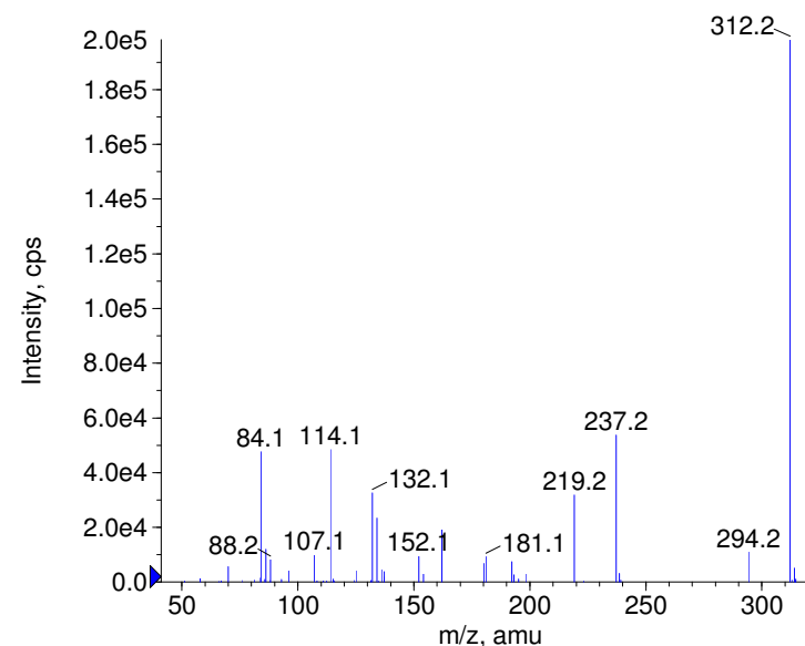
+ Xantinol Prec(312.0) CE(99.0) RT(0.9)
