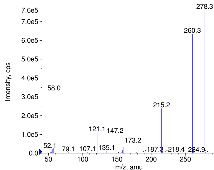
+ Venlafaxine Prec(278.0) CE(50.0) RT(0.7)
