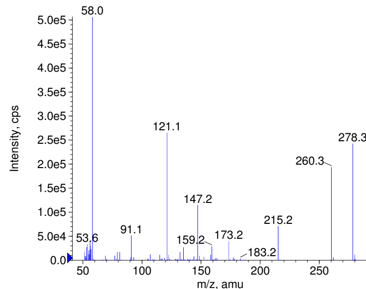
+ Venlafaxine Prec(278.0) CE(99.0) RT(0.7)
