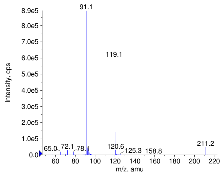
+ Tripelennamine Prec(256.0) CE(50.0) RT(0.9)
