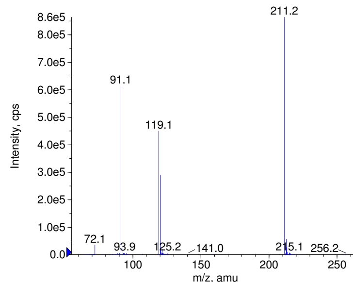
+ Tripelennamine Prec(256.0) CE(99.0) RT(0.9)
