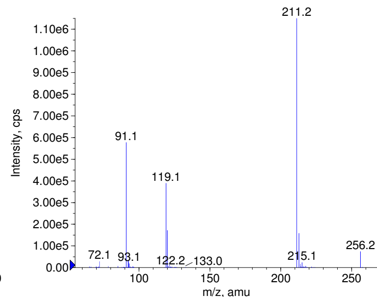
+ Tripelennamine Prec(256.0) CE(99.0) RT(0.9)
