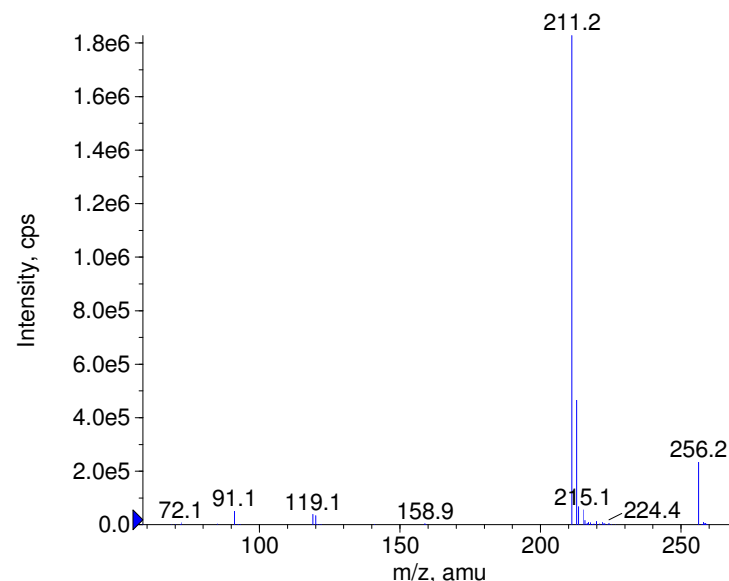
+ Tripelennamine Prec(256.0) CE(50.0) RT(0.9)
