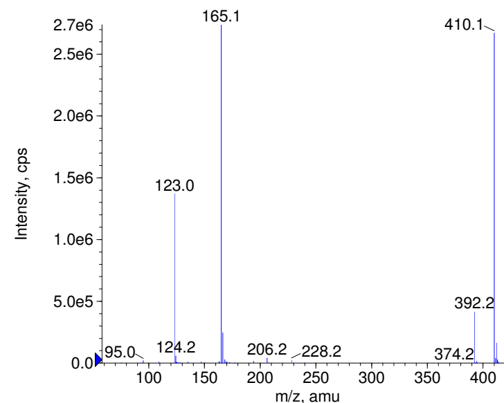
■ + Trifluoperidol Prec(410.0) CE(99.0) RT(0.8)
