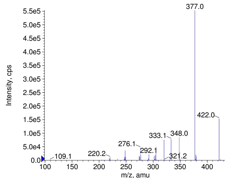
■ + Topotecan Prec(422.0) CE(99.0) RT(0.9)
