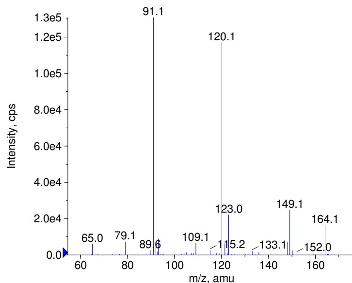
■ + Tolnaftate Prec(308.0) CE(50.0) RT(0.8)
