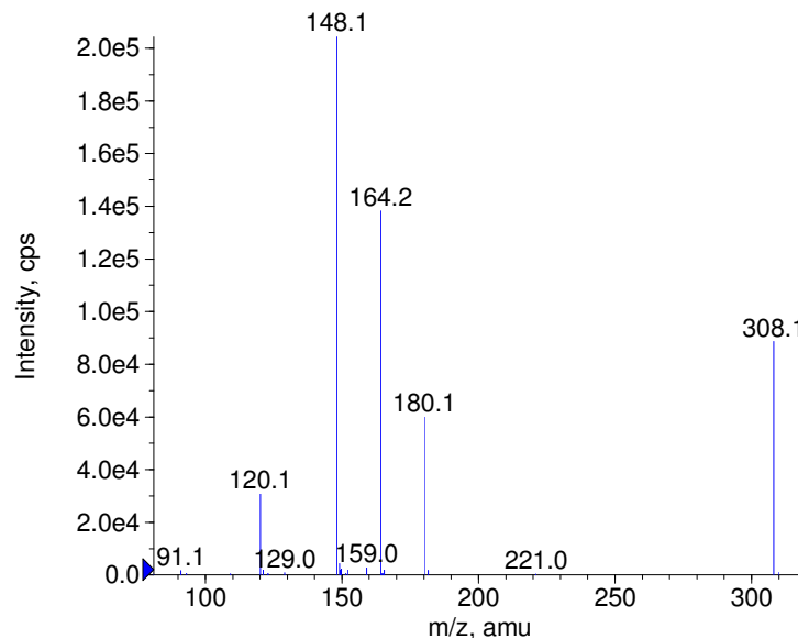
■ + Tolnaftate Prec(308.0) CE(50.0) RT(0.8)
