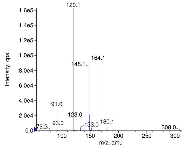
■ + Tolnaftate Prec(308.0) CE(99.0) RT(0.9)
