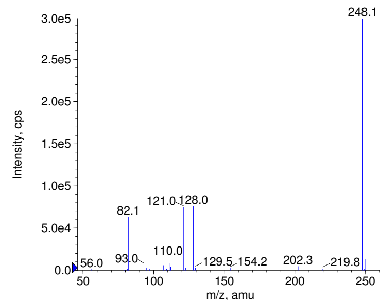
+ Tinidazole Prec(248.0) CE(99.0) RT(0.9)
