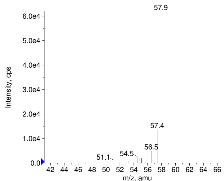
■ - Thiopental Prec(241.0) CE(-50.0) RT(0.9)
