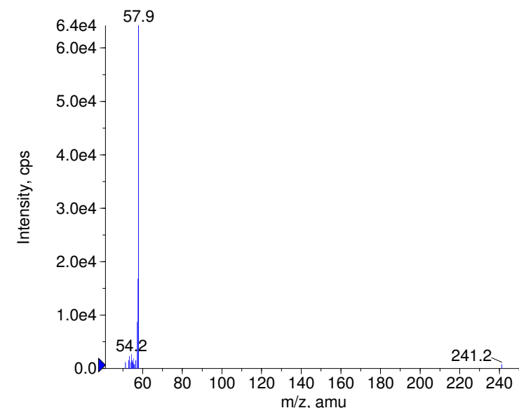
■ - Thiopental Prec(241.0) CE(-99.0) RT(0.9)
