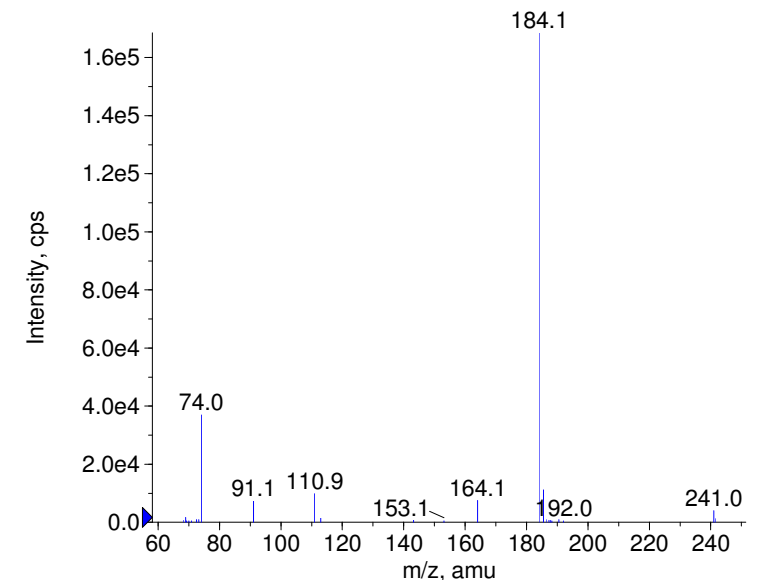
+ Thiazaflurone Prec(241.0) CE(99.0) RT(0.9)
