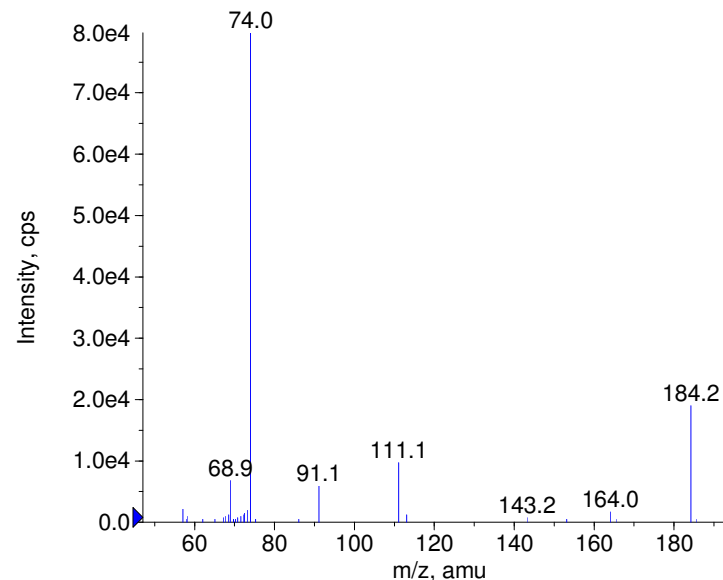
+ Thiazaflurone Prec(241.0) CE(50.0) RT(0.9)
