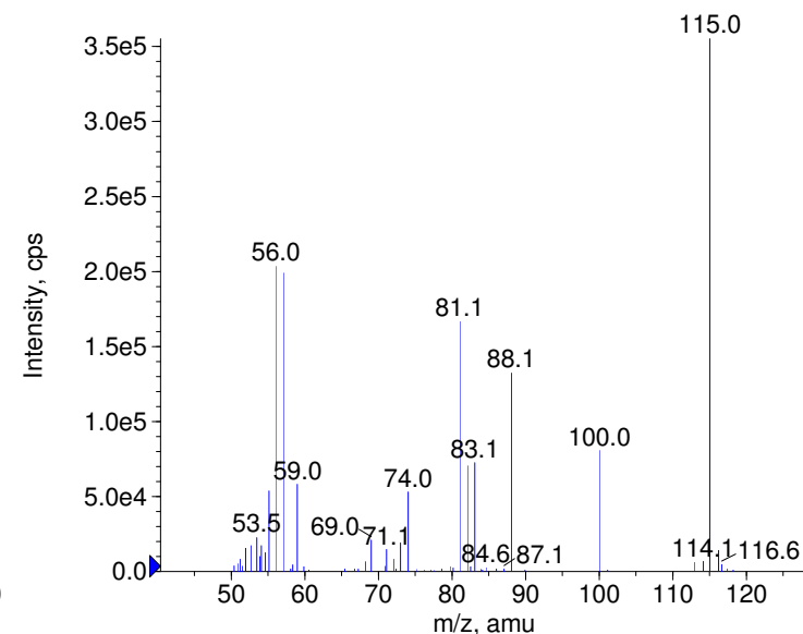
+ Thiamazole Prec(115.0) CE(99.0) RT(1.1)
