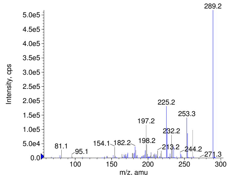
+ Tetrazepam Prec(289.0) CE(99.0) RT(1.4)
