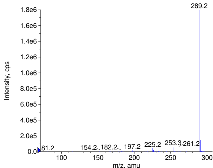
+ Tetrazepam Prec(289.0) CE(50.0) RT(1.3)
