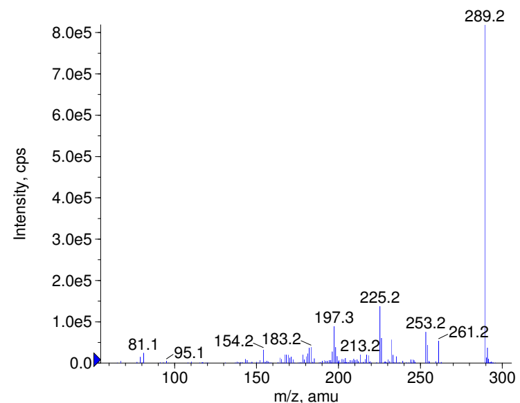
+ Tetrazepam Prec(289.0) CE(99.0) RT(1.4)
