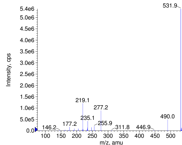
+ Terconazole Prec(532.0) CE(99.0) RT(0.7)
