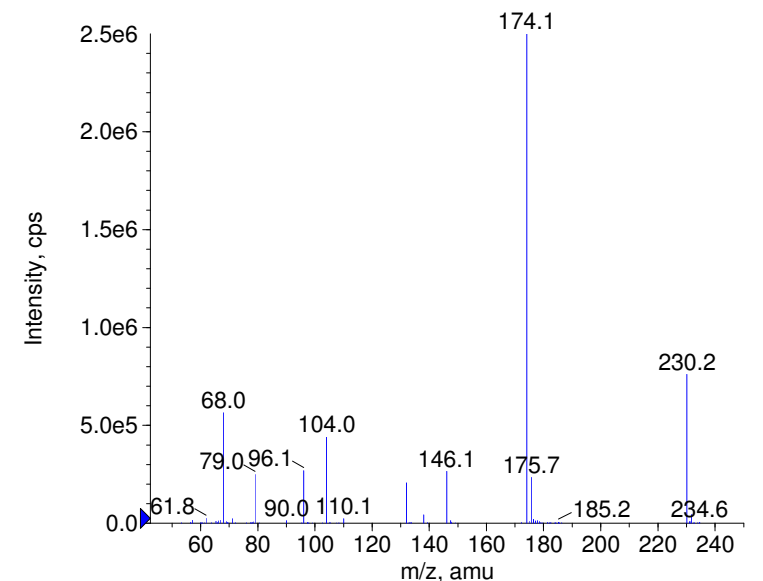
+ Terbutylazine Prec(230.0) CE(99.0) RT(1.2)
