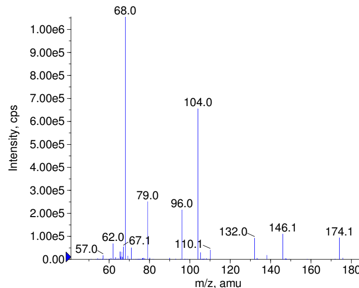
+ Terbutylazine Prec(230.0) CE(50.0) RT(1.1)
