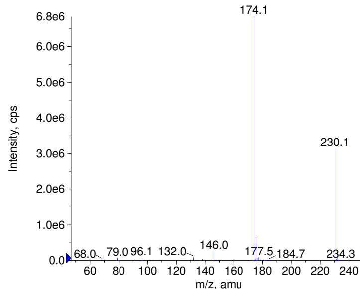
+ Terbutylazine Prec(230.0) CE(50.0) RT(1.1)
