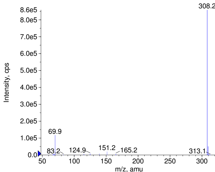
+ Tebuconazole Prec(308.0) CE(50.0) RT(0.9)
