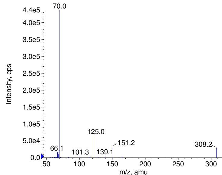
+ Tebuconazole Prec(308.0) CE(99.0) RT(0.9)
