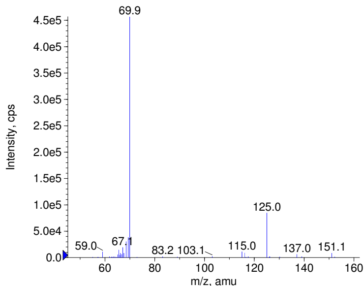
+ Tebuconazole Prec(308.0) CE(50.0) RT(0.9)
