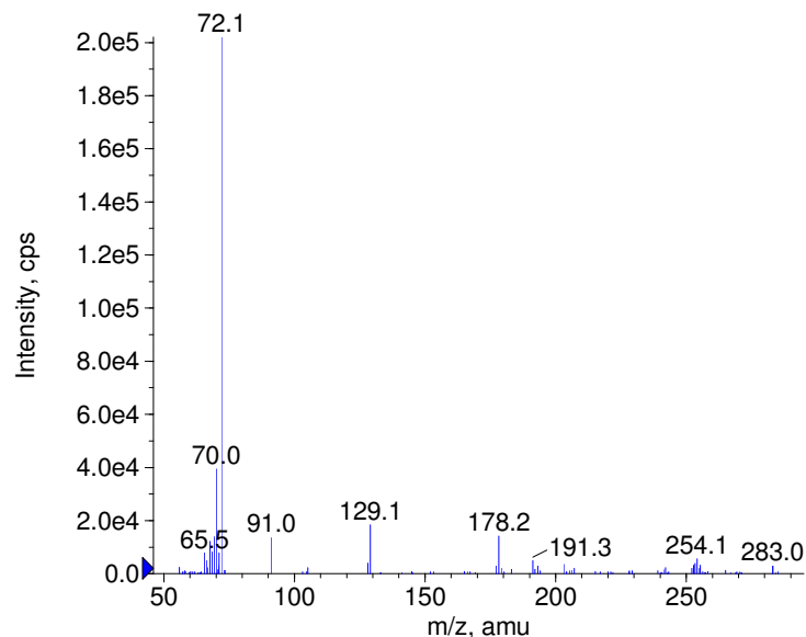
+ Tamoxifen Prec(372.0) CE(50.0) RT(0.9)
