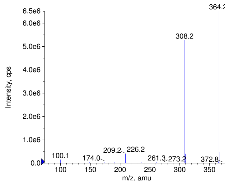
+ Talinolol Prec(364.0) CE(50.0) RT(0.8)
