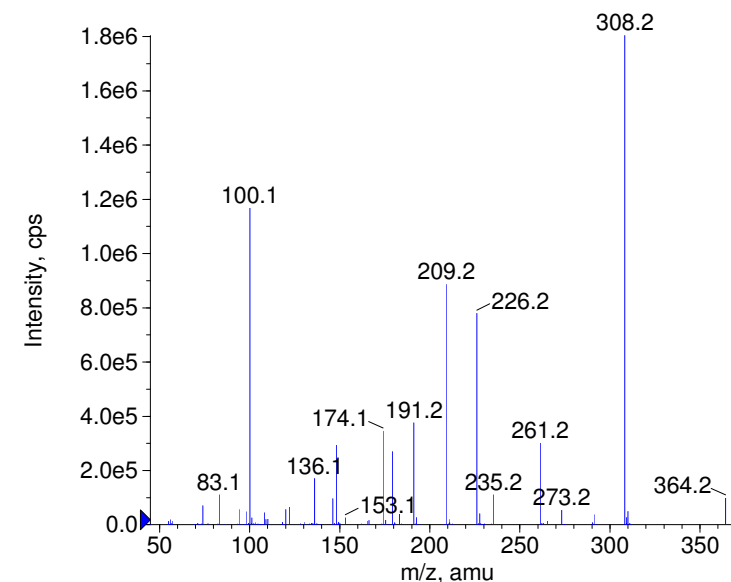
+ Talinolol Prec(364.0) CE(99.0) RT(0.8)
