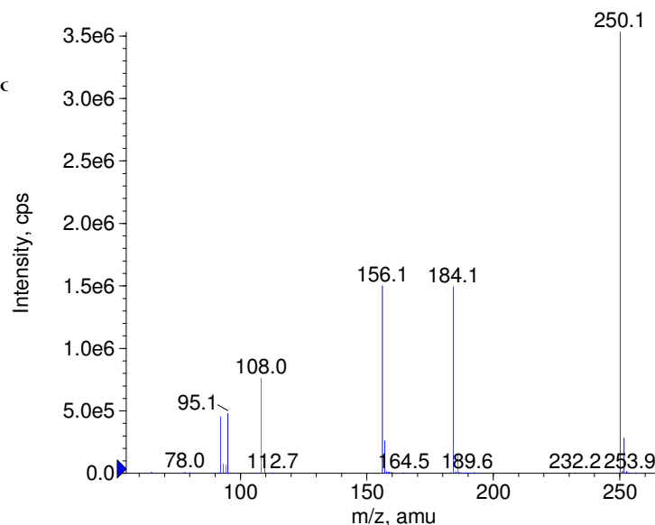
■ + Sulfapyridine Prec(250.0) CE(50.0) RT(0.8)
