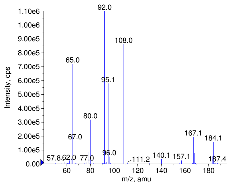
■ + Sulfapyridine Prec(250.0) CE(50.0) RT(0.8)
