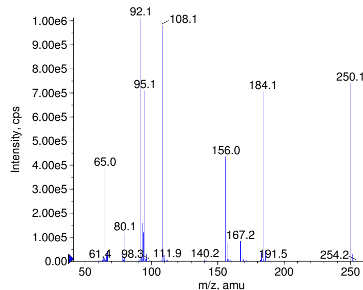
■ + Sulfapyridine Prec(250.0) CE(99.0) RT(0.8)
