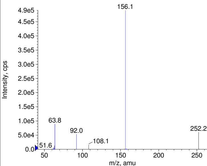
■ - Sulfamethoxazole Prec(252.0) CE(-99.0) RT(0.9)
