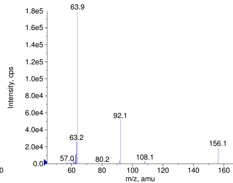
■ - Sulfamethoxazole Prec(252.0) CE(-50.0) RT(0.8)
