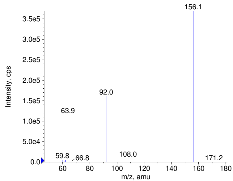
■ - Sulfamethoxazole Prec(252.0) CE(-35.0) RT(0.8)
