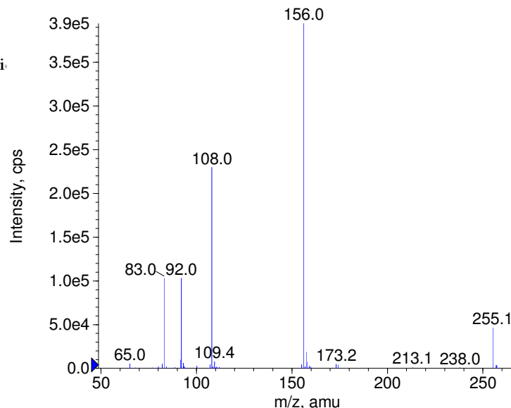
+ Sulfadiazine Prec(255.0) CE(50.0) RT(0.8)
