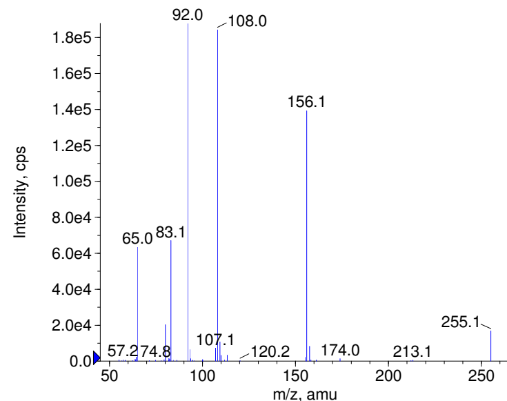
+ Sulfadiazine Prec(255.0) CE(99.0) RT(0.8)
