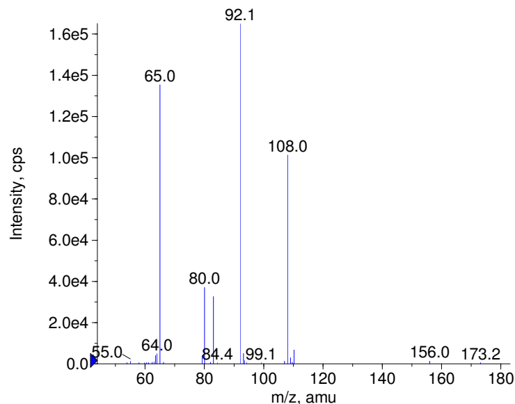
+ Sulfadiazine Prec(255.0) CE(50.0) RT(0.8)
