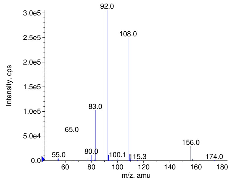
+ Sulfadiazine Prec(255.0) CE(99.0) RT(0.8)
