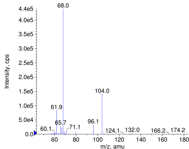
+ Simazine Prec(202.0) CE(50.0) RT(0.9)
