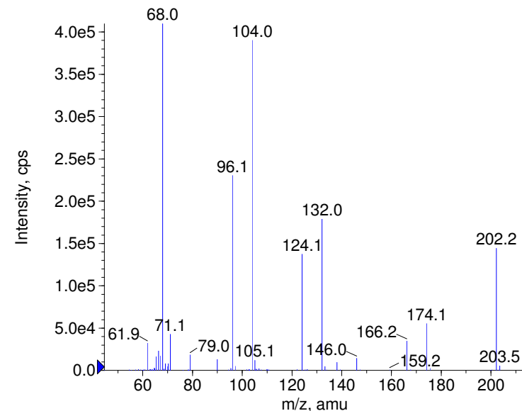
+ Simazine Prec(202.0) CE(99.0) RT(0.9)
