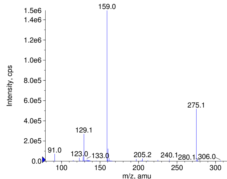
+ Sertraline Prec(306.0) CE(99.0) RT(0.8)
