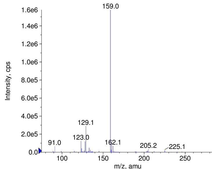
+ Sertraline Prec(306.0) CE(50.0) RT(0.8)
