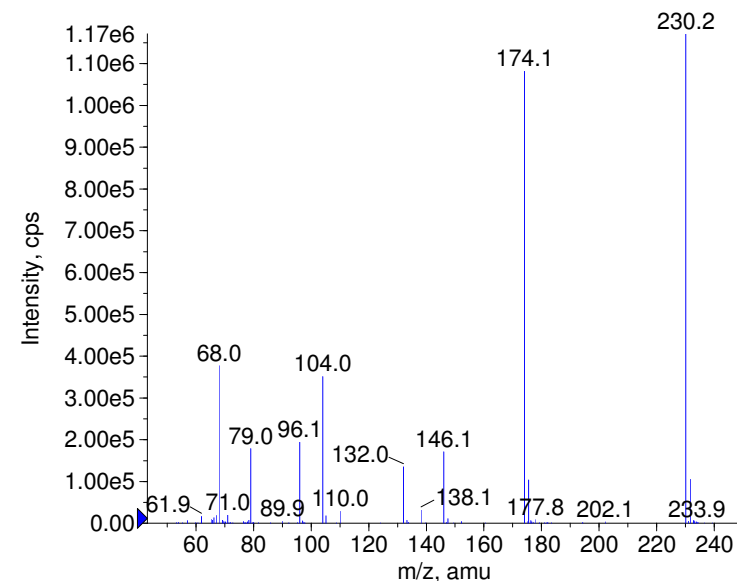
+ Sebuthylazine Prec(230.0) CE(99.0) RT(1.1)
