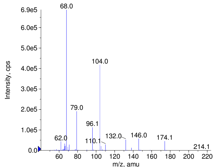
+ Sebuthylazine Prec(230.0) CE(50.0) RT(1.1)
