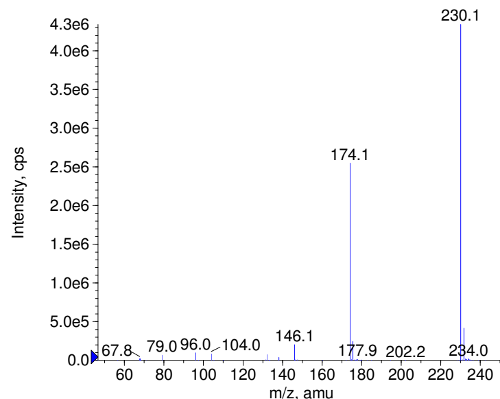
+ Sebuthylazine Prec(230.0) CE(50.0) RT(1.1)
