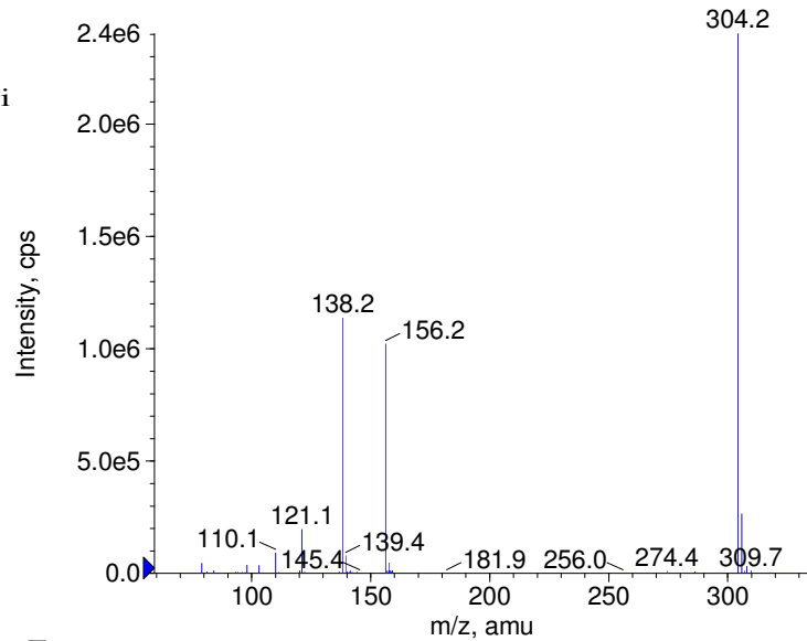
■ + Scopolamine Prec(304.0) CE(50.0) RT(0.7)
