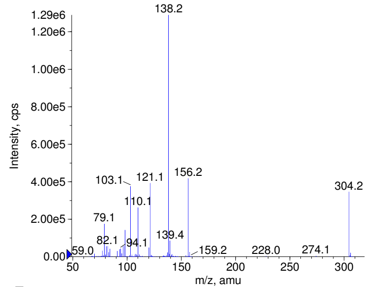
■ + Scopolamine Prec(304.0) CE(99.0) RT(0.8)
