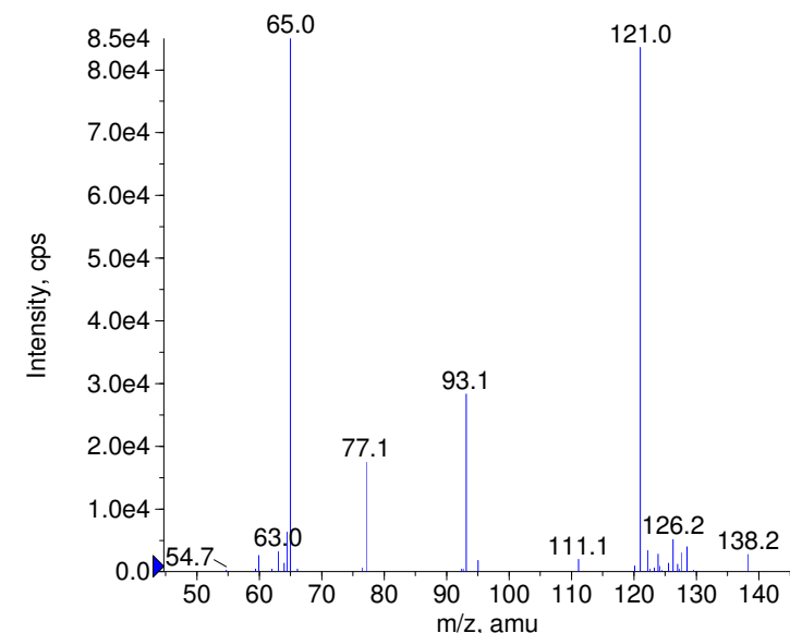
+ Salicylamide Prec(138.0) CE(99.0) RT(1.0)
