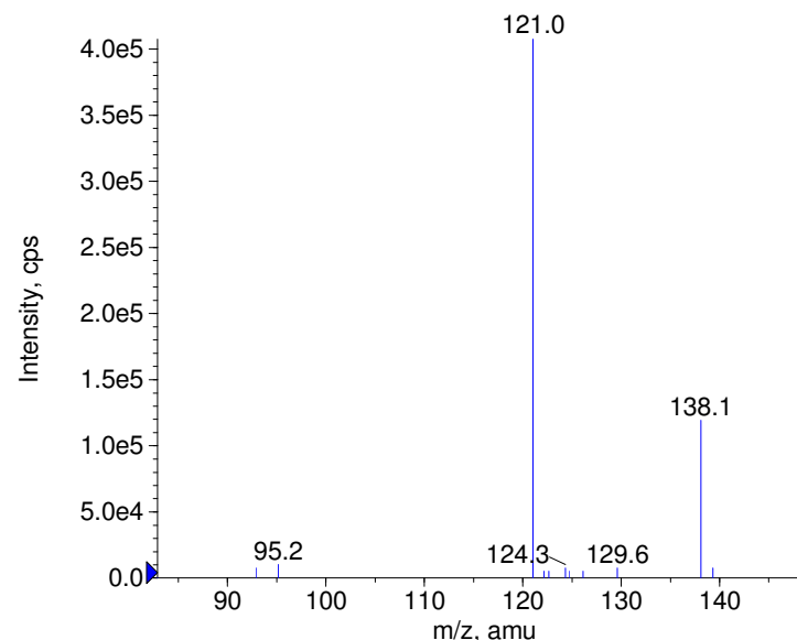
+ Salicylamide Prec(138.0) CE(50.0) RT(1.0)
