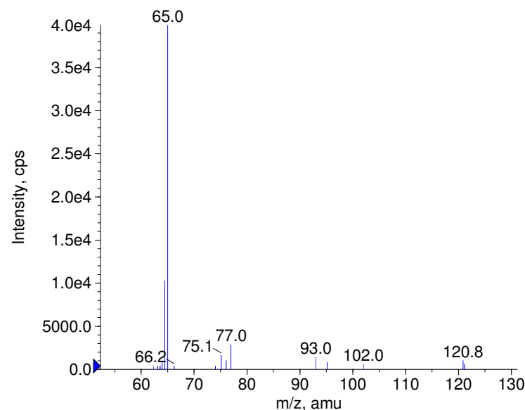
+ Salicylamide Prec(138.0) CE(50.0) RT(1.0)
