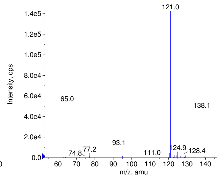
+ Salicylamide Prec(138.0) CE(99.0) RT(1.0)
