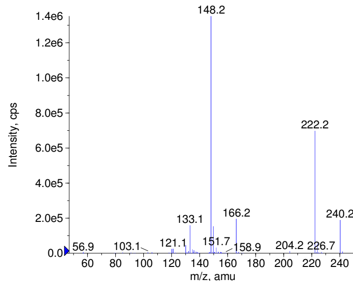
+ Salbutamol Prec(240.0) CE(50.0) RT(0.8)
