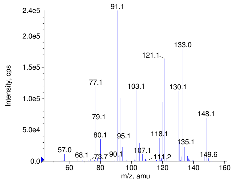
+ Salbutamol Prec(240.0) CE(50.0) RT(0.8)
