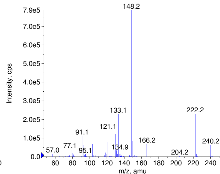
+ Salbutamol Prec(240.0) CE(99.0) RT(0.8)
