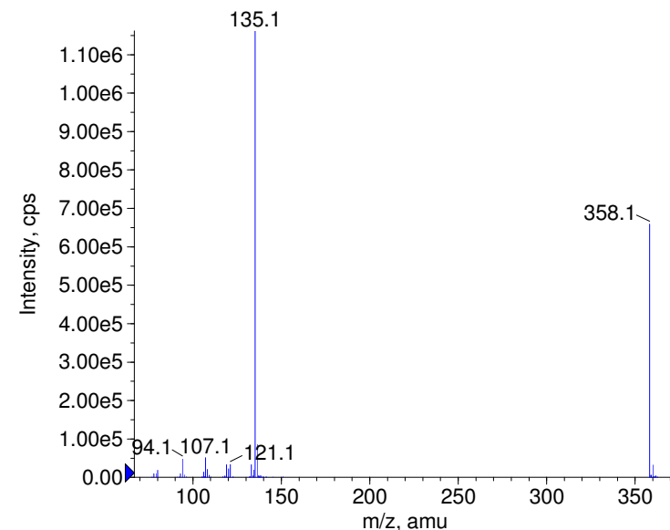
+ Rosiglitazon Prec(358.0) CE(99.0) RT(0.7)
