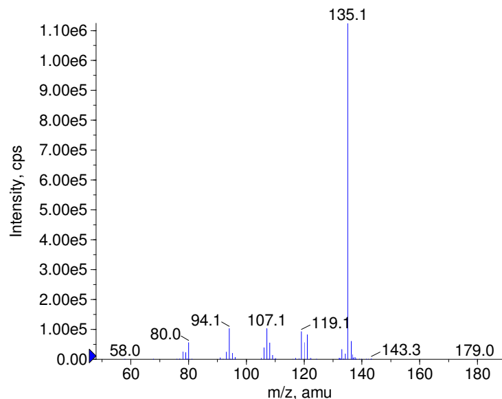
+ Rosiglitazon Prec(358.0) CE(50.0) RT(0.7)
