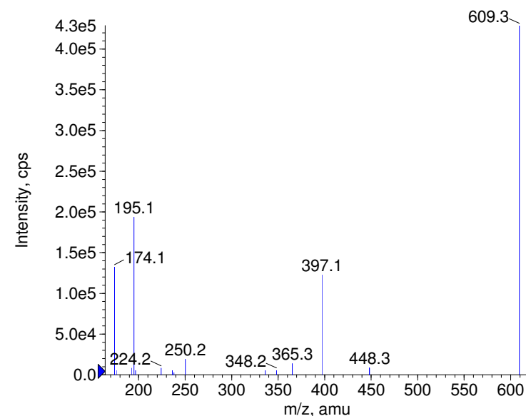
■ + Reserpin Prec(609.0) CE(99.0) RT(0.9)
