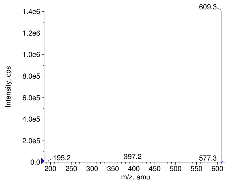
■ + Reserpin Prec(609.0) CE(50.0) RT(0.9)
