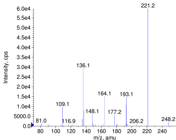
+ Reproterol Prec(390.0) CE(50.0) RT(0.7)
