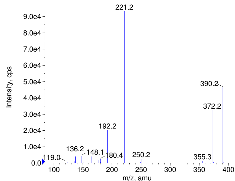
+ Reproterol Prec(390.0) CE(99.0) RT(0.7)
