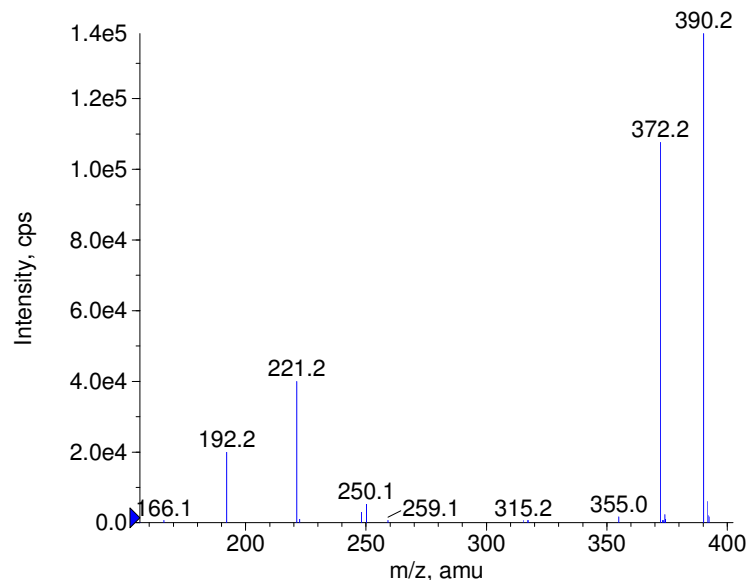
+ Reproterol Prec(390.0) CE(50.0) RT(0.7)
