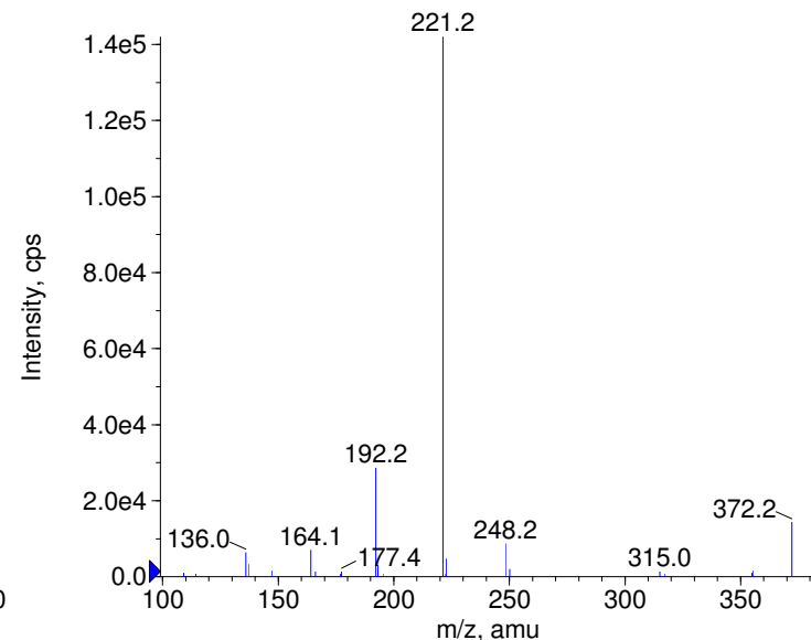
+ Reproterol Prec(390.0) CE(99.0) RT(0.7)
