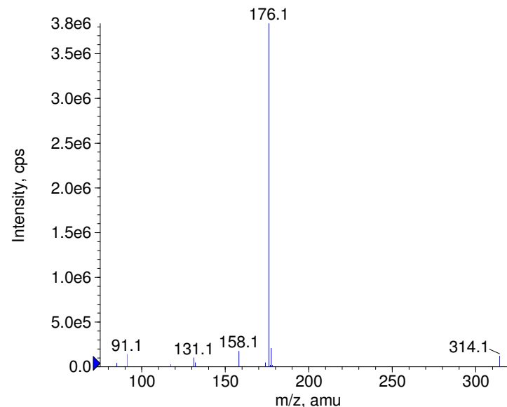
+ Reboxetine Prec(314.0) CE(50.0) RT(1.0)
