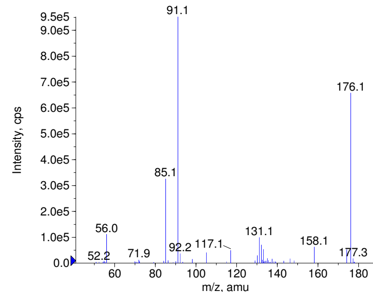
+ Reboxetine Prec(314.0) CE(99.0) RT(1.0)
