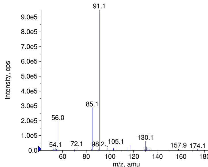
+ Reboxetine Prec(314.0) CE(50.0) RT(1.0)
