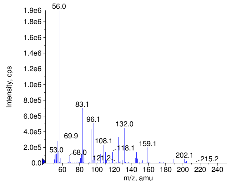
+ Ramifenazone Prec(246.0) CE(99.0) RT(0.9)
