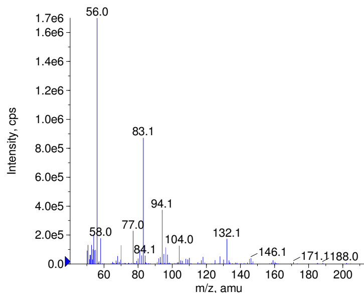
+ Ramifenazone Prec(246.0) CE(50.0) RT(0.9)
