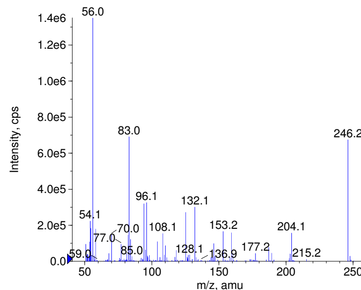
+ Ramifenazone Prec(246.0) CE(99.0) RT(0.9)
