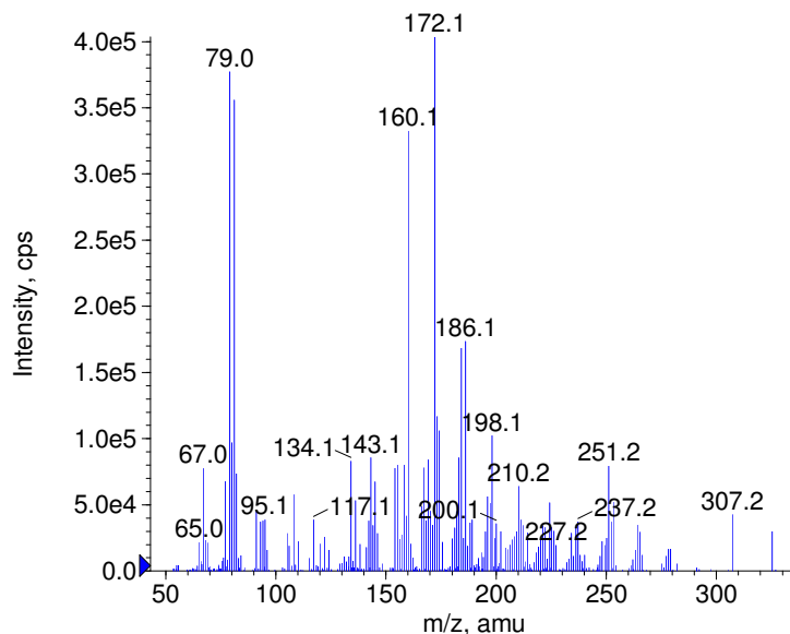
+ Quinine Prec(325.0) CE(50.0) RT(0.7)
