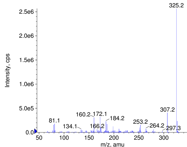
+ Quinine Prec(325.0) CE(99.0) RT(0.7)
