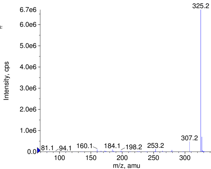
+ Quinine Prec(325.0) CE(50.0) RT(0.7)
