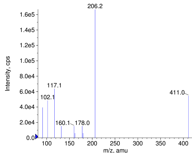
+ Quinaprilat Prec(411.0) CE(99.0) RT(0.9)
