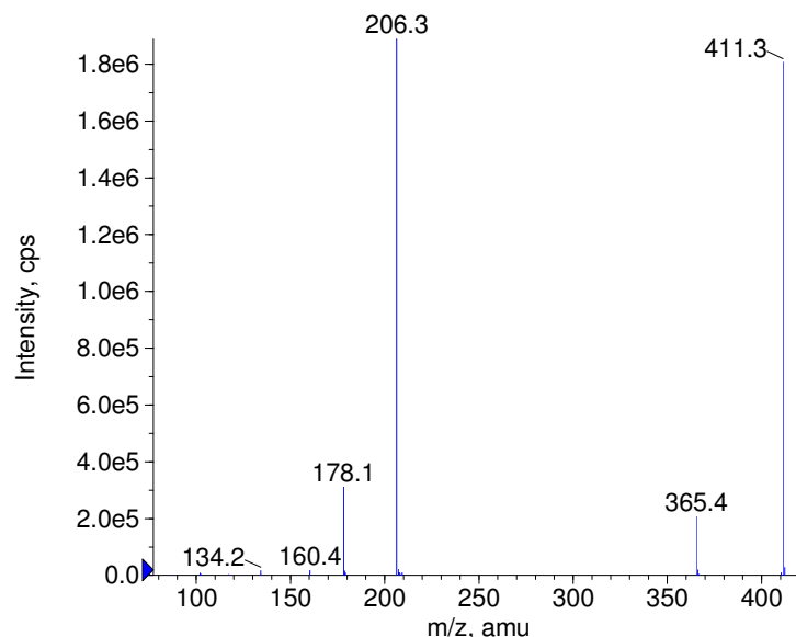
+ Quinaprilat Prec(411.0) CE(50.0) RT(0.9)
