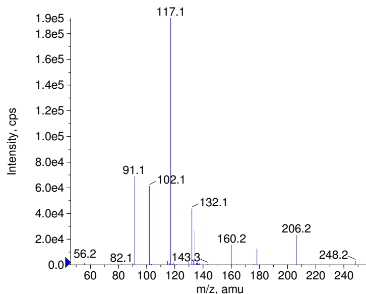
+ Quinaprilat Prec(411.0) CE(50.0) RT(0.9)
