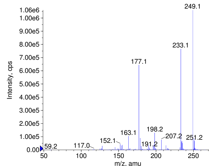
+ Pyrimethamine Prec(249.0) CE(99.0) RT(0.9)
