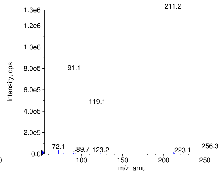
+ Pyribenzamine Prec(256.0) CE(99.0) RT(0.9)
