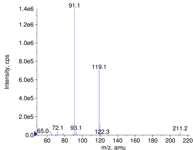
+ Pyribenzamine Prec(256.0) CE(50.0) RT(0.9)
