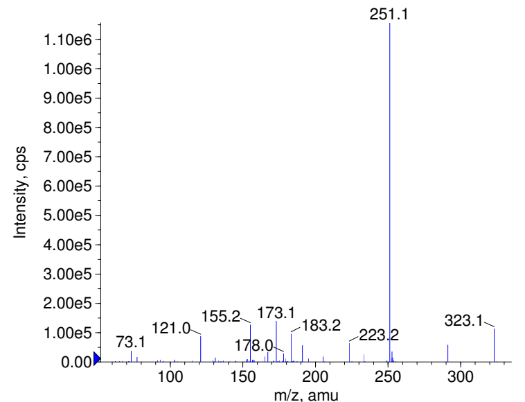
+ Pyranocoumarin Prec(323.0) CE(99.0) RT(3.4)
