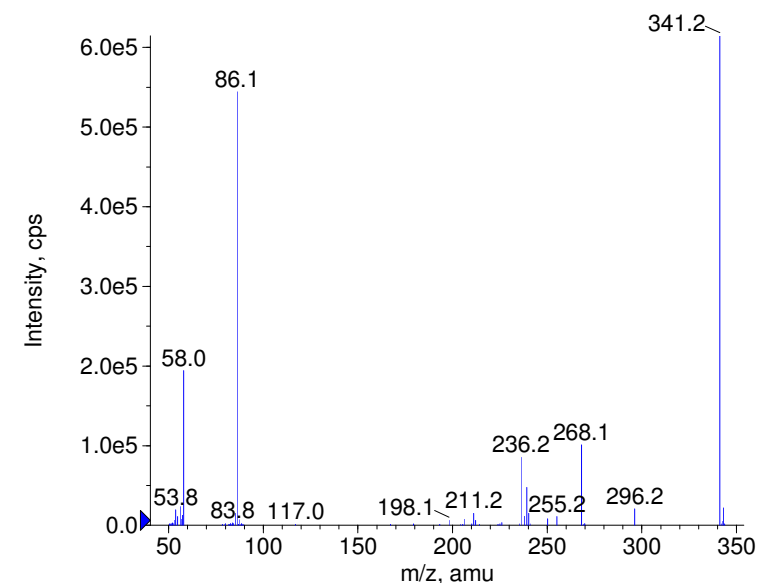
+ Propionylpromazine Prec(341.0) CE(99.0) RT(0.7)
