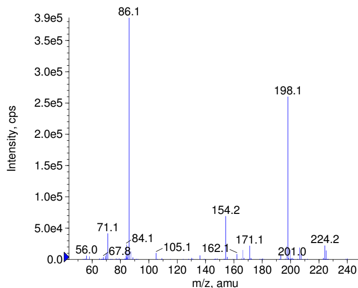
+ Promethazine Prec(285.0) CE(50.0) RT(0.8)
