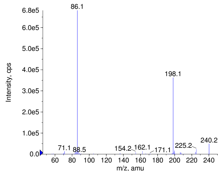
+ Promethazine Prec(285.0) CE(99.0) RT(0.8)
