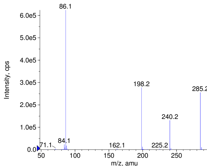
+ Promethazine Prec(285.0) CE(50.0) RT(0.8)
