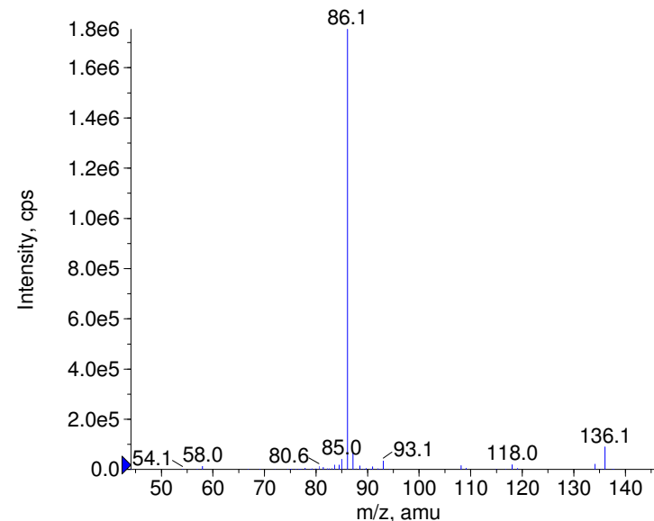
+ Prilocaine Prec(221.0) CE(99.0) RT(0.8)
