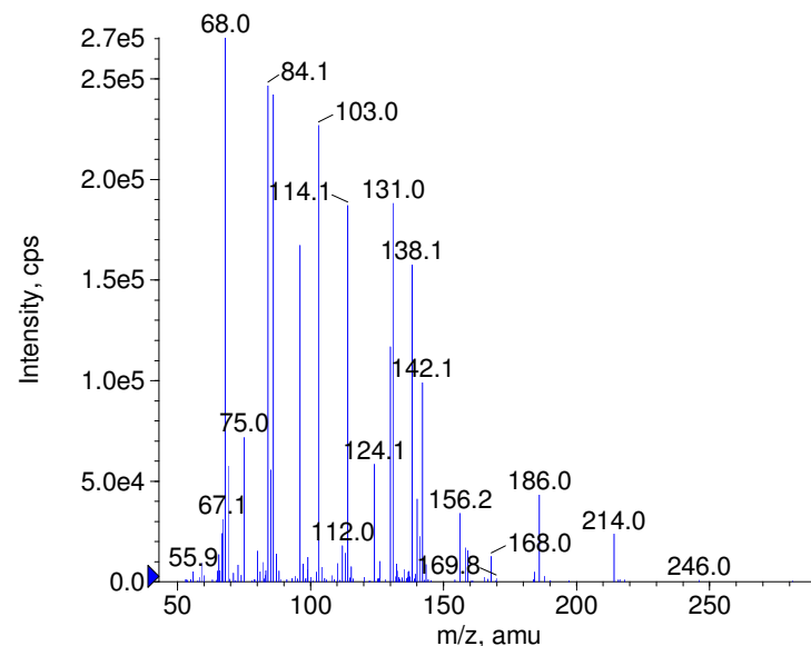
+ Piprozolin Prec(299.0) CE(50.0) RT(1.2)
