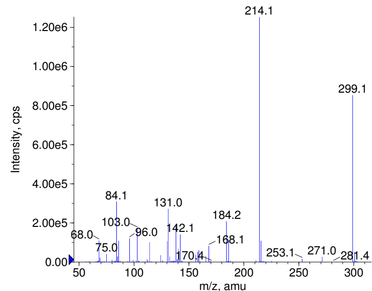
+ Piprozolin Prec(299.0) CE(99.0) RT(1.2)
