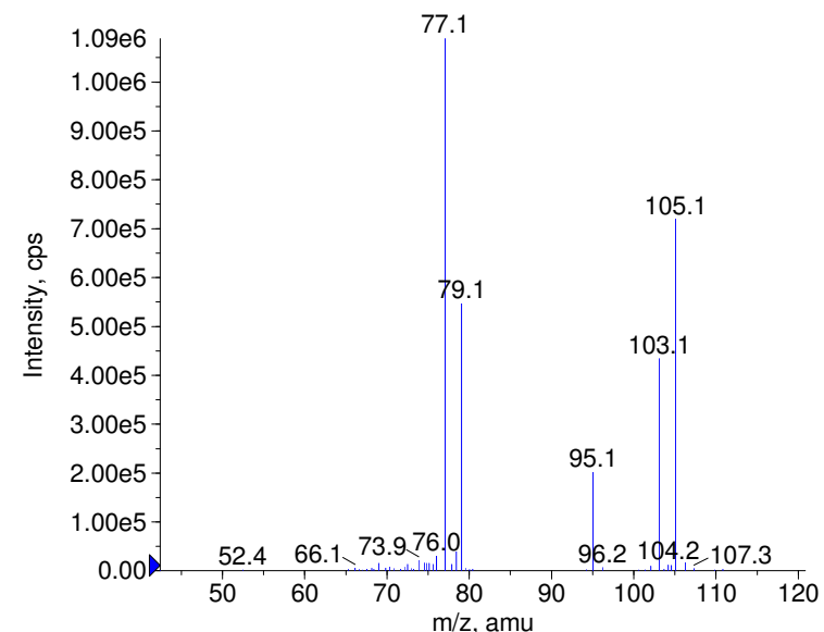
+ Phenethylamin Prec(122.0) CE(99.0) RT(1.0)
