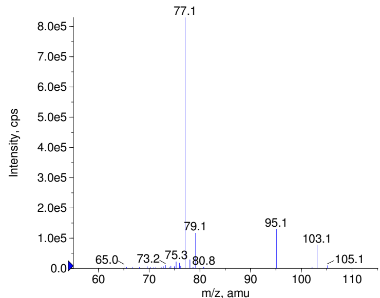
+ Phenethylamin Prec(122.0) CE(50.0) RT(1.0)
