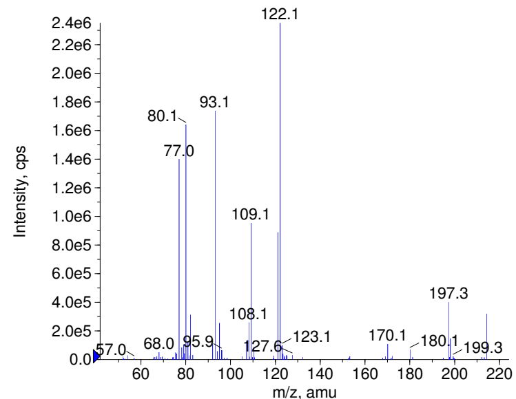
■ + Phenazopyridine Prec(214.0) CE(99.0) RT(0.9)
