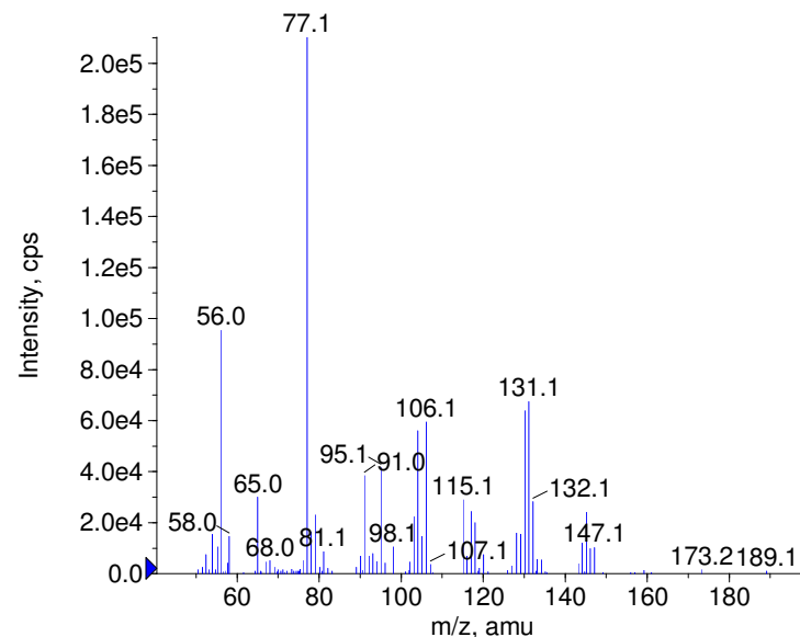
+ Phenazone Prec(189.0) CE(50.0) RT(0.9)
