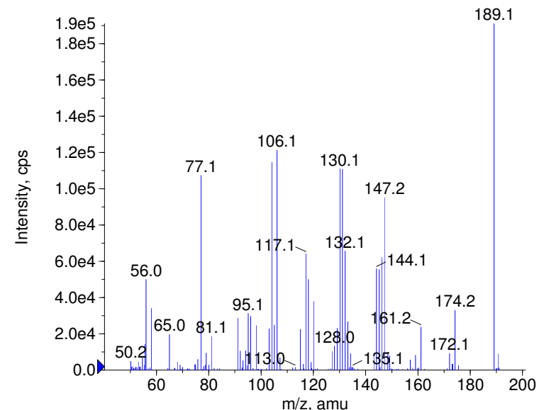
+ Phenazone Prec(189.0) CE(99.0) RT(0.9)
