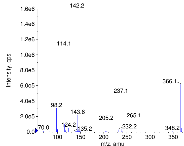
+ Periciazine Prec(366.0) CE(99.0) RT(0.8)
