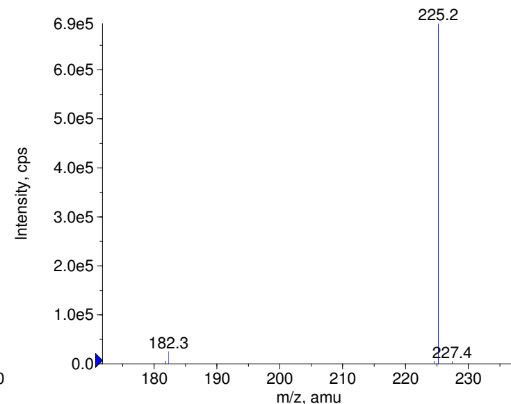
■ - Pentobarbital Prec(225.0) CE(-99.0) RT(0.9)
