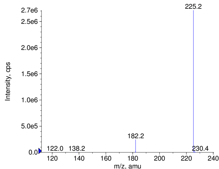
■ - Pentobarbital Prec(225.0) CE(-50.0) RT(0.9)
