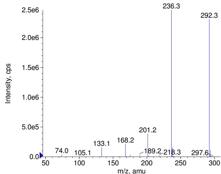
+ Penbutolol Prec(292.0) CE(50.0) RT(0.9)
