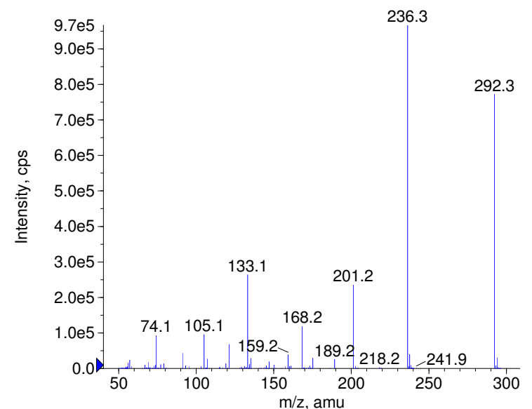
+ Penbutolol Prec(292.0) CE(99.0) RT(0.9)
