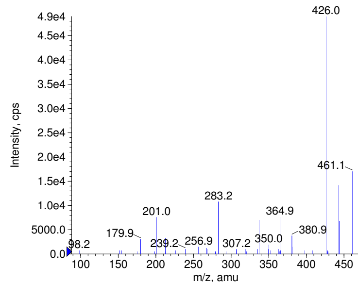
■ + Oxytetracycline Prec(461.0) CE(99.0) RT(0.9)
