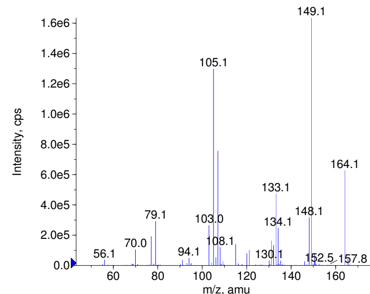
+ Oxilofrine Prec(182.0) CE(99.0) RT(0.8)
