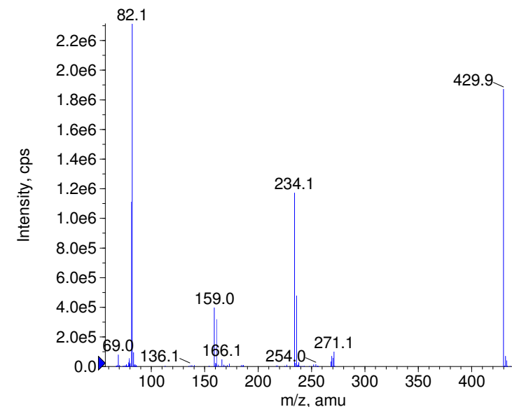
+ Oxiconazole Prec(430.0) CE(99.0) RT(1.6)
