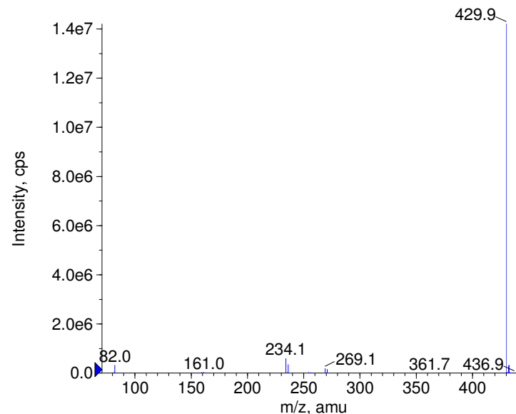
+ Oxiconazole Prec(430.0) CE(50.0) RT(1.6)
