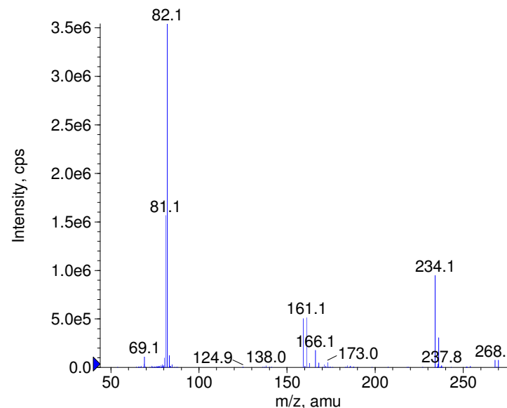
+ Oxiconazole Prec(430.0) CE(50.0) RT(1.6)
